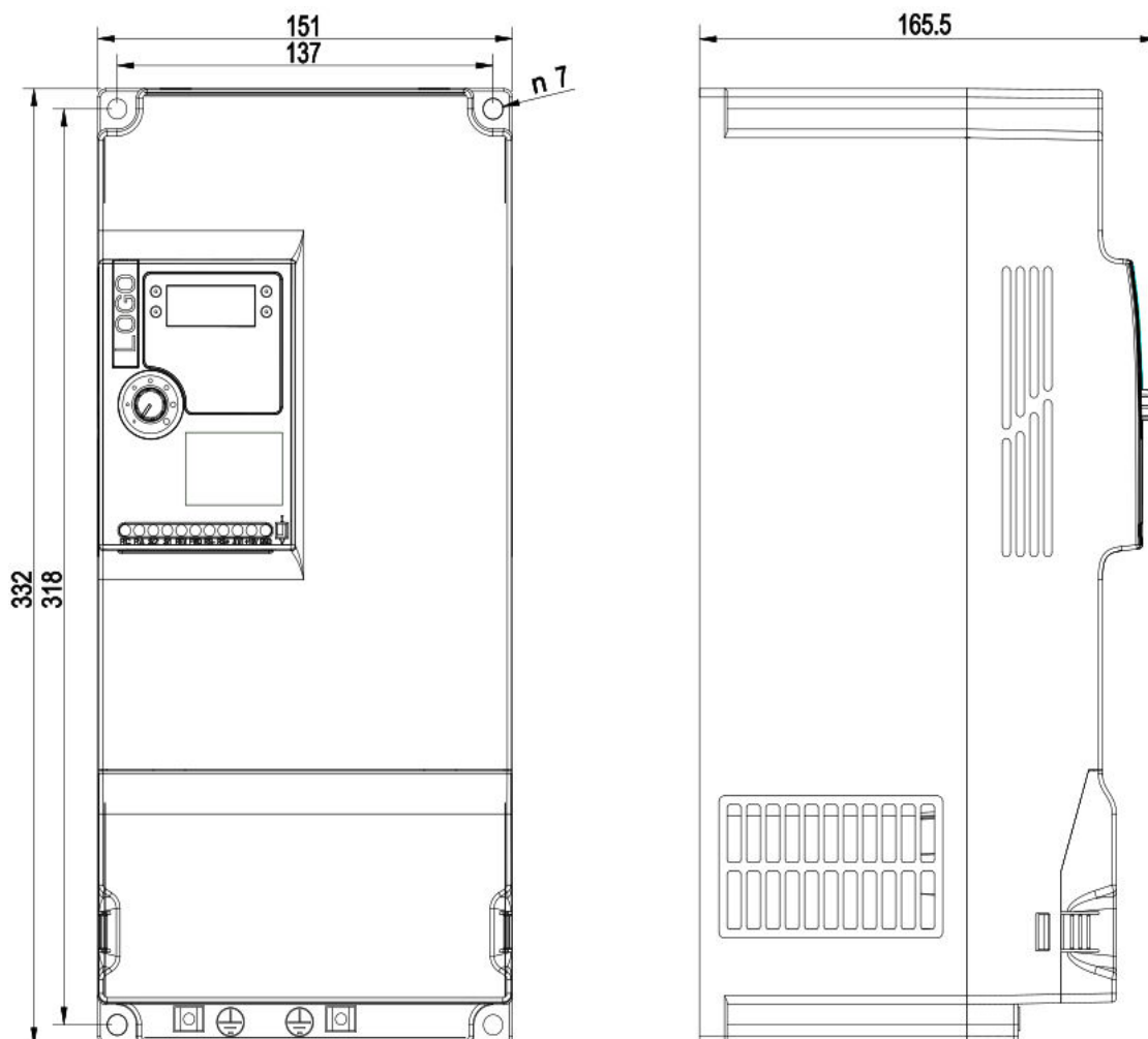
Rozmerový výkres A550 PLUS - 15kW 4T0150
