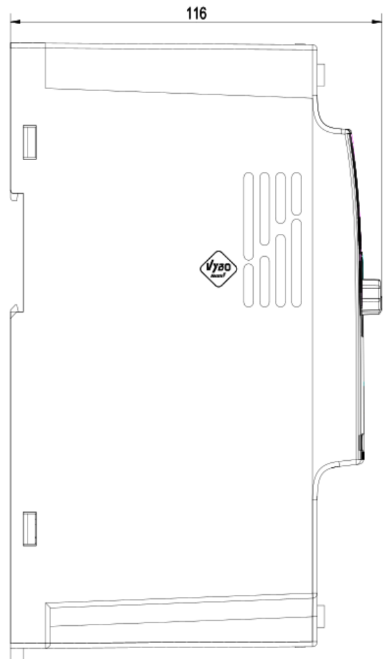
Rozmerový výkres A550 PLUS - 3kW 2S0030
