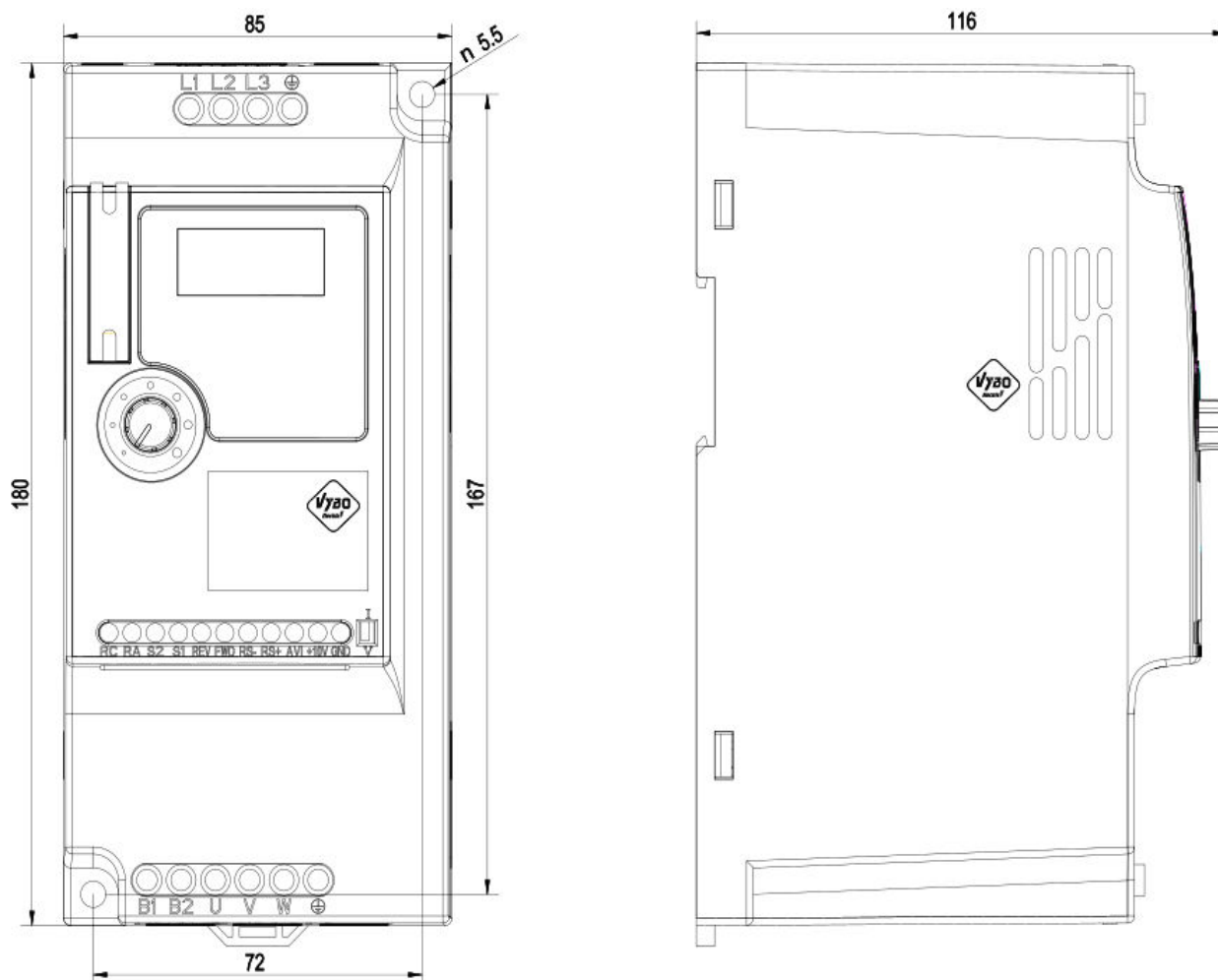
Rozmerový výkres A550 PLUS - 4kW 4T0040
