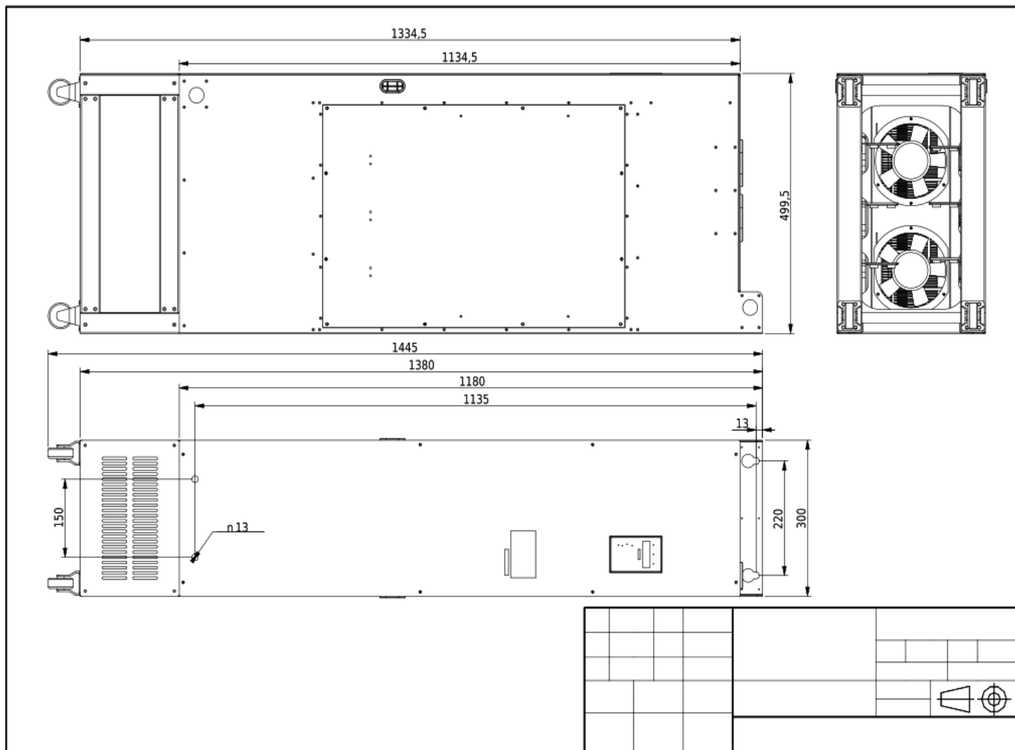
Rozmerový výkres V800 - 185kW 4T1850
