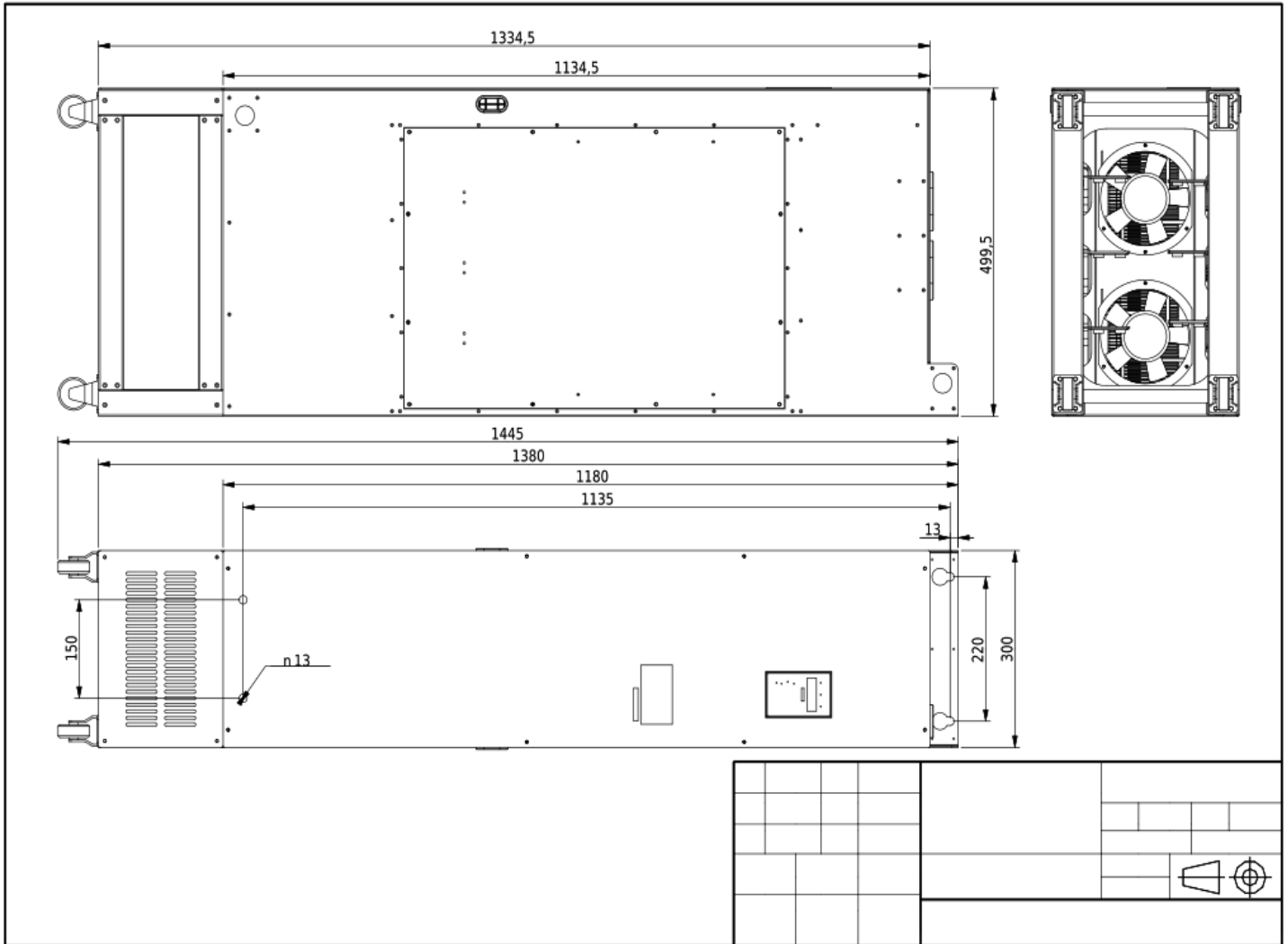
Rozmerový výkres V800 - 200kW 4T2000
