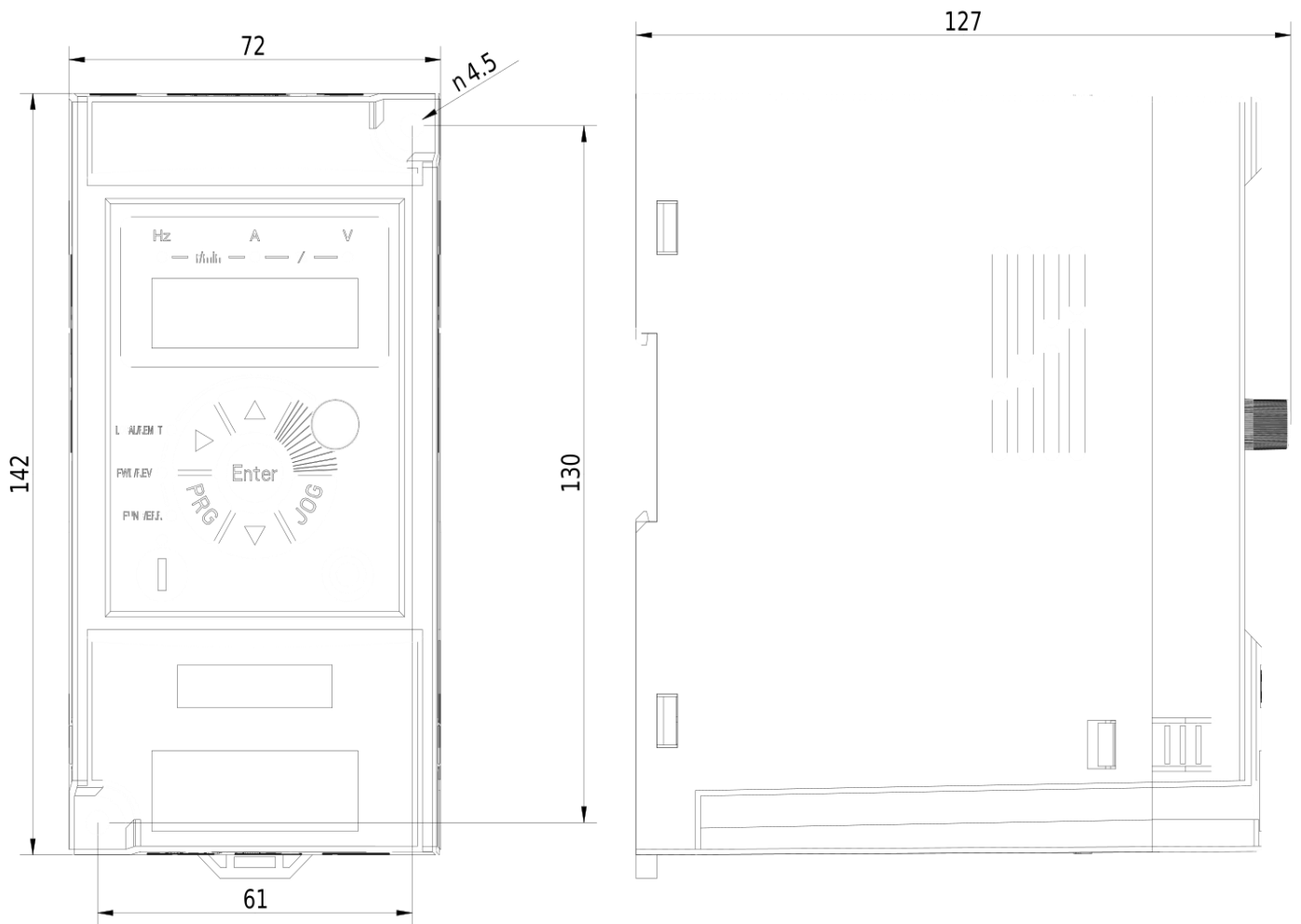
Rozmerový výkres V900 - 1,5kW 2S0015
