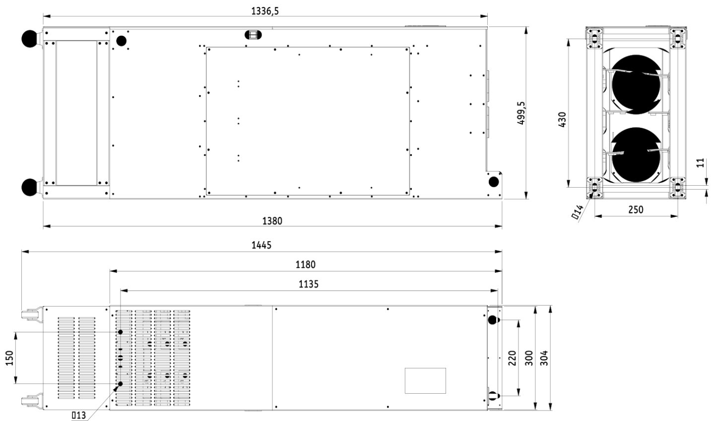
Rozmerový výkres V900 - 200kW 4T2000
