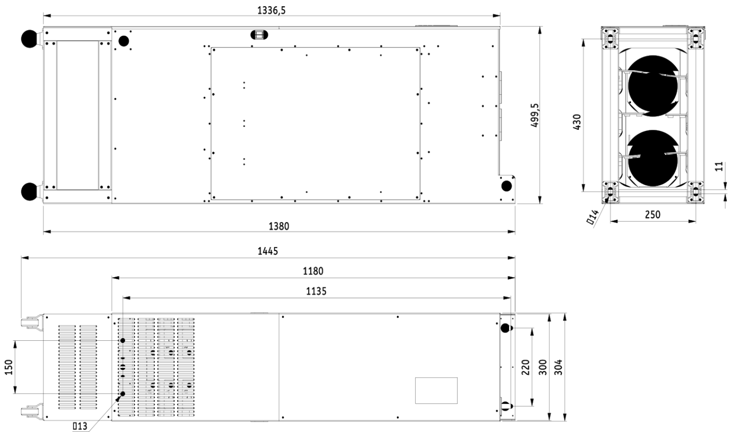
Rozmerový výkres V900 - 220kW 4T2200
